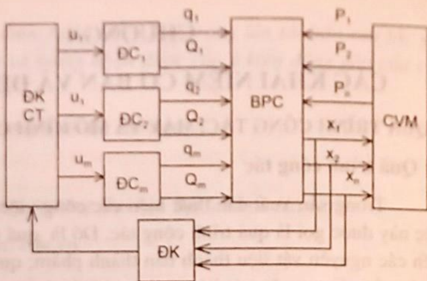
Hình 1.2 Sơ đồ máy nhiều động cơ
